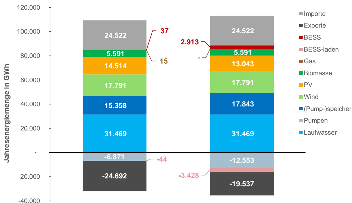
Abbildung 1: Jahresenergiemenge je Technologie bei uneingeschränkter Abregelung von PV und Wind (links) und bei maximal 10% Abregelung je Zeitschritt (rechts).
