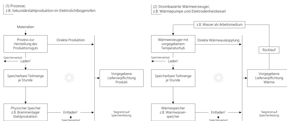
Abbildung 1: Konzeptionelle Darstellung der Funktionalität des Flexibilitätsmoduls für Prozesse(1) und strombasierte Wärmeerzeuger(2)
