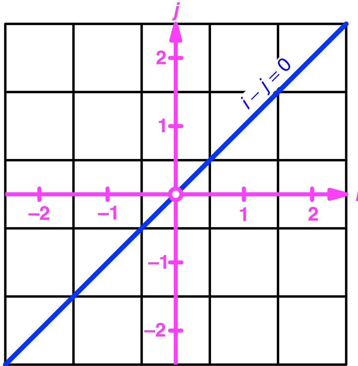
Geradengleichung
