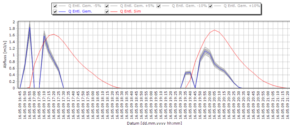
Ereignis 032 Entlastung
