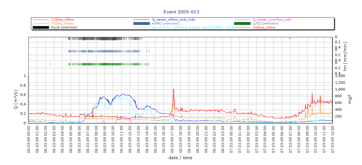
Abbildung 3-10 Darstellung der Abflussganglinien und Niederschlag Ereignis 013
