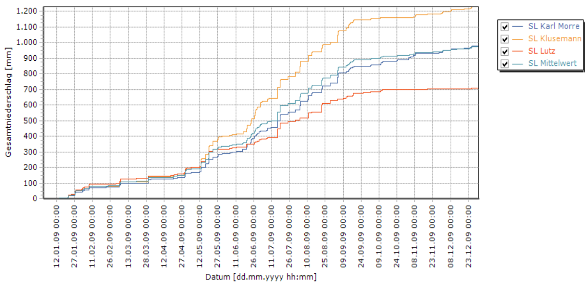
Abbildung 3-1 Vergleich Jahresganglinie und Mittelwert (2009)
