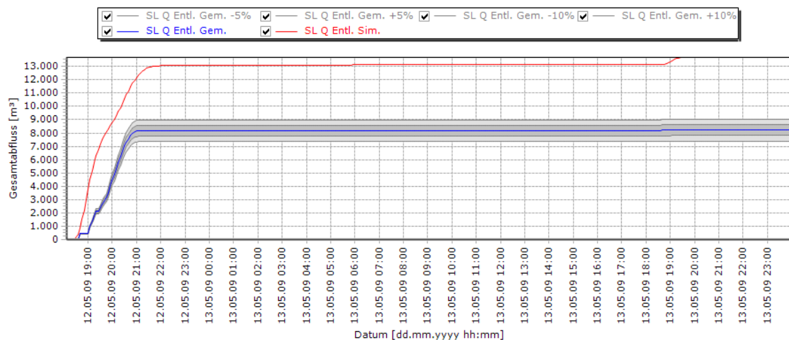
Ereignis 028_029 Summenlinien Entlastung
