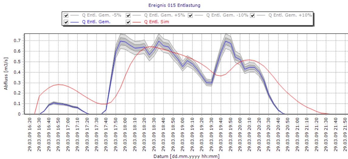
Abbildung 4-7 Ganglinie Ereignis 015
