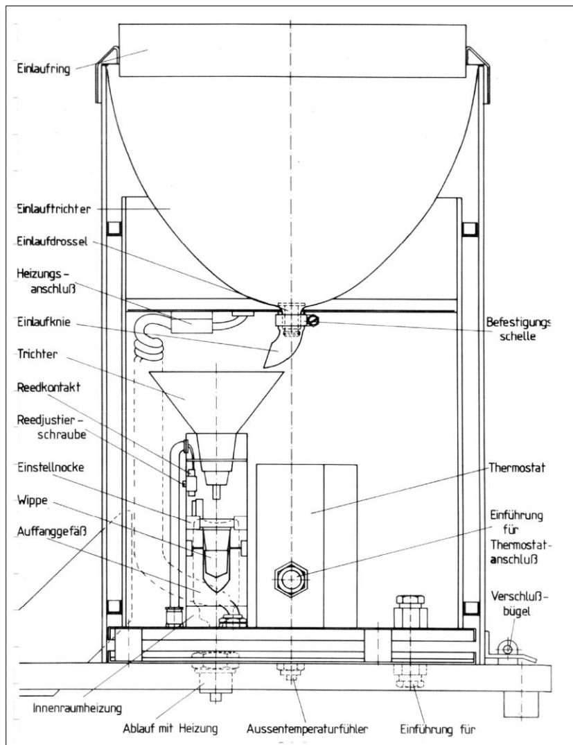
Abbildung 2-11: Detaillierter Aufbau einer Niederschlagswippe (Thaler, 2004)
