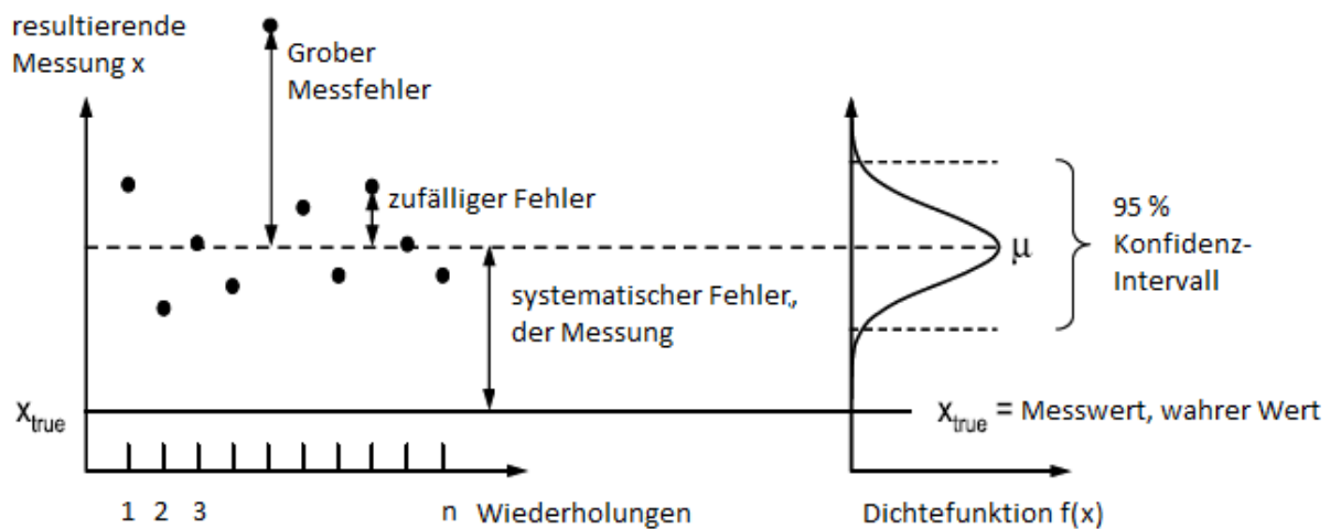
Abbildung 2-4 Übersicht der Fehlerarten aus Gujer, W. (2008, nach Thomann (2002), modifiziert)
