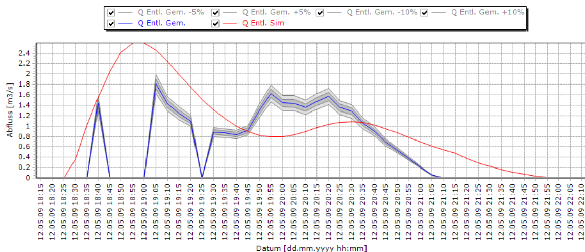
Ereignis 028_029 Entlastung
