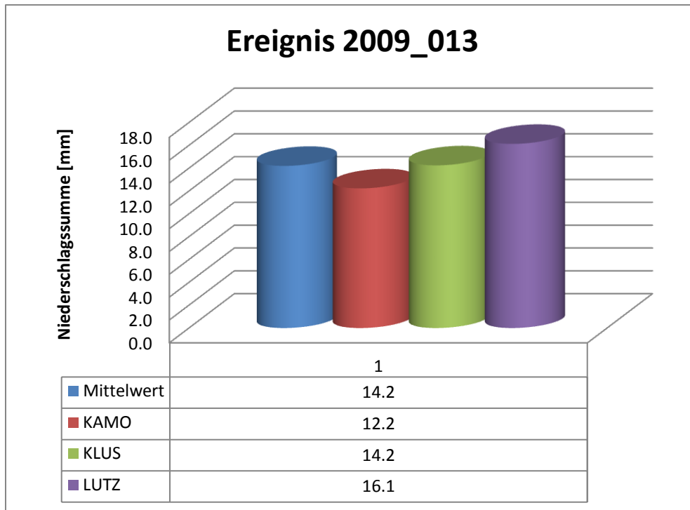
Abbildung 3-11 Vergleich Niederschlagssummen und Mittelwert Ereignis 2009_013
