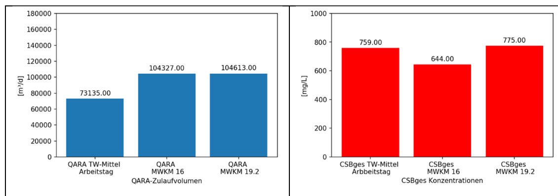
Abbildung 5-37: Vergleich der Q_{ARA} -Zulaufmengen und CSB_{ges} -Konzentrationen vom Trockenwettermittel „Arbeitstag“ mit dem Mischwasserereignis MWKM 16 und MWKM 19.2
