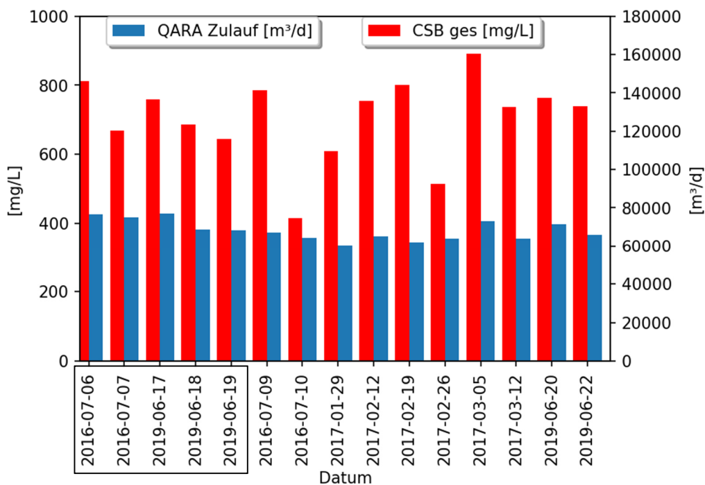
Abbildung 5-6: CSB ges und zugehörige Tagezuflussmengen Q ARA der gemessenen Trockenwettertage. Links umrandet an Arbeitstagen; Rest an Wochenend- und Feiertagen
