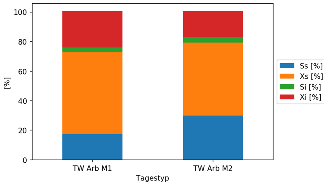
Abbildung 5-22: Vergleich der relativen Anteile der CSB-Fraktionen am CSB_{ges} der Trockenwettermittel „Arbeitstag“ M1 vs. M3
