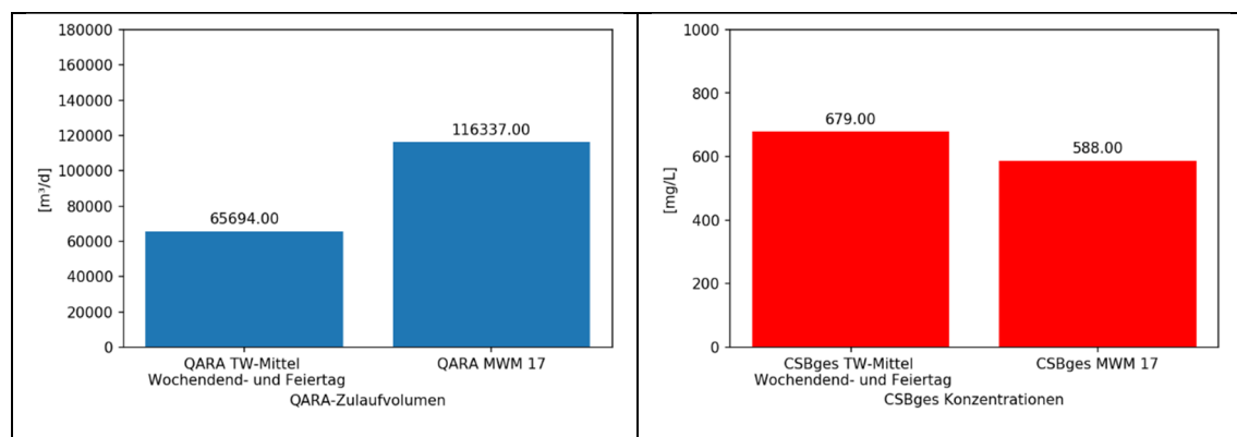
Abbildung 5-34: Vergleich der Q ARA -Zulaufmengen und CSB ges -Konzentrationen vom Trockenwettermittel „Wochenend- und Feiertag“ mit dem Mischwasserereignis MWM 17
