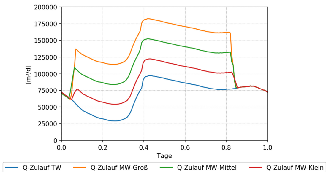
Abbildung 5-44: Zuläufe des Trockenwetter und der drei Mischwasserszenarien (10-Minutenintervalle)
