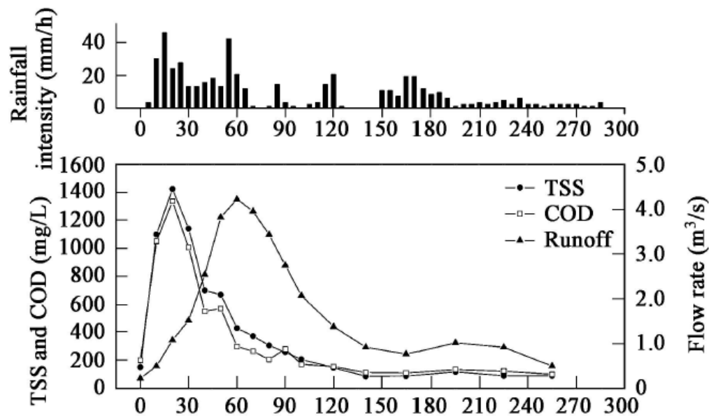
Abbildung 3-5: COD und TSS Konzentrationsspitzen zu Beginn des Abflusses angesichts eines Niederschlagsereignisses (Li et al., 2007)
