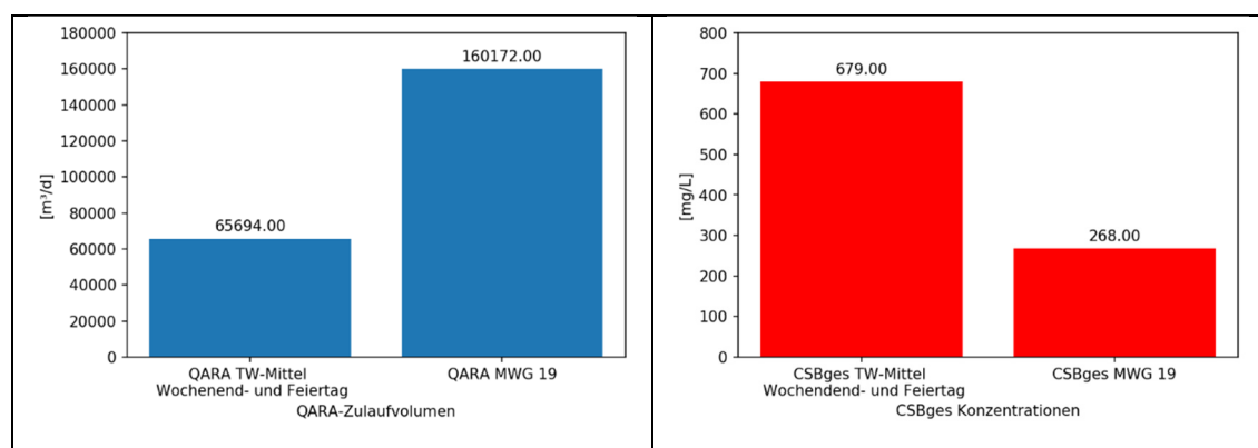
Abbildung 5-31: Vergleich der Q ARA -Zulaufmengen und CSB ges -Konzentrationen vom Trockenwettermittel „Wochenend- und Feiertag“ mit dem Mischwasserereignis MWG 19
