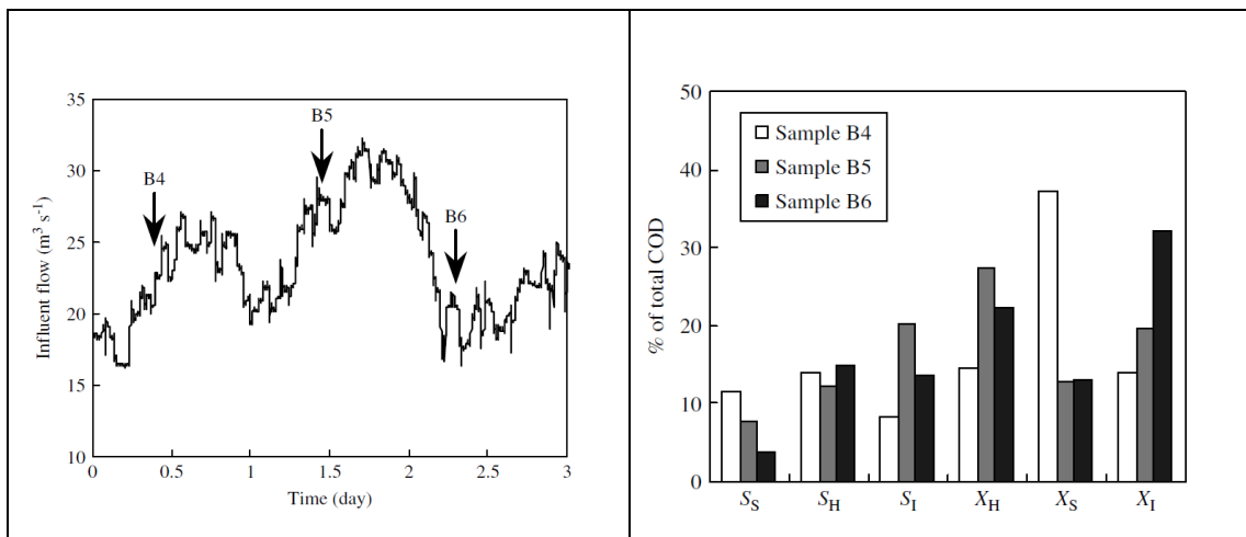
Abbildung 3-4: Zufluss zur Kläranlage „Bailonggang“ während des Taifuns und die analytisch bestimmten CSB-Fractionen von drei Abwasserproben unterschiedlicher Zeitpunkte (Zhou et al., 2008)
