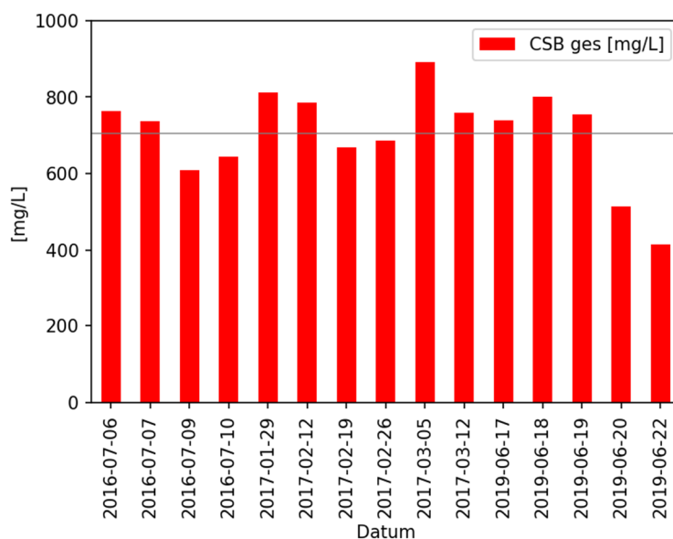
Abbildung 5-4: CSB ges -Konzentrationen der Trockenwettertage: CSB-Mittel = 705 mg/L
