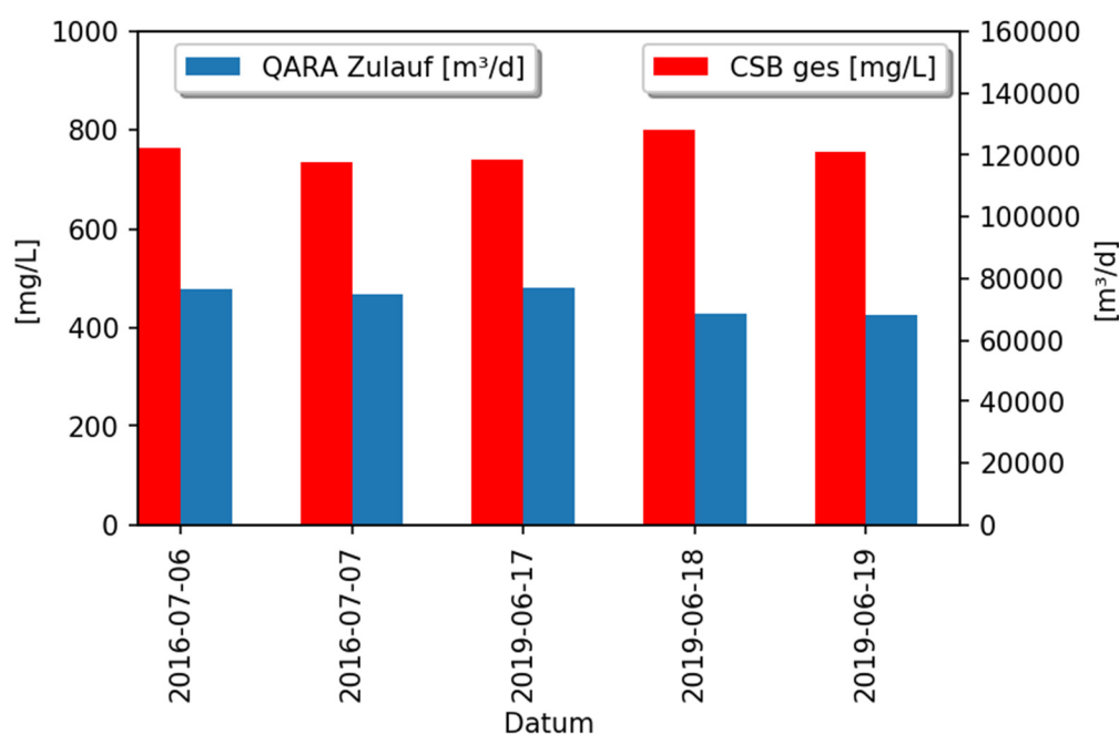
Abbildung 5-9: Q_{ARA} -Zulaufmenge und CSB ges -Konzentrationen der Trockenwettertage für das Trockenwettermittel des Tagestyps „Arbeitstag“
