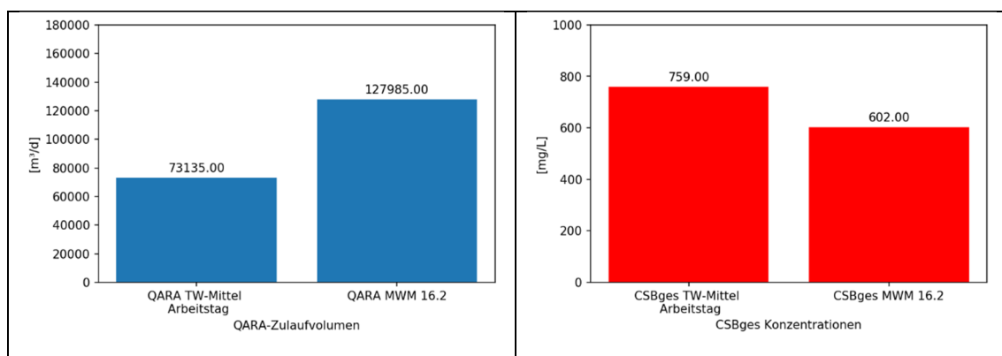
Abbildung 5-40. Vergleich der QARA-Zulaufmengen und CSB ges -Konzentrationen vom Trockenwettermittel „ Arbeitstag “ mit dem Mischwasserereignis MWM 16.2
