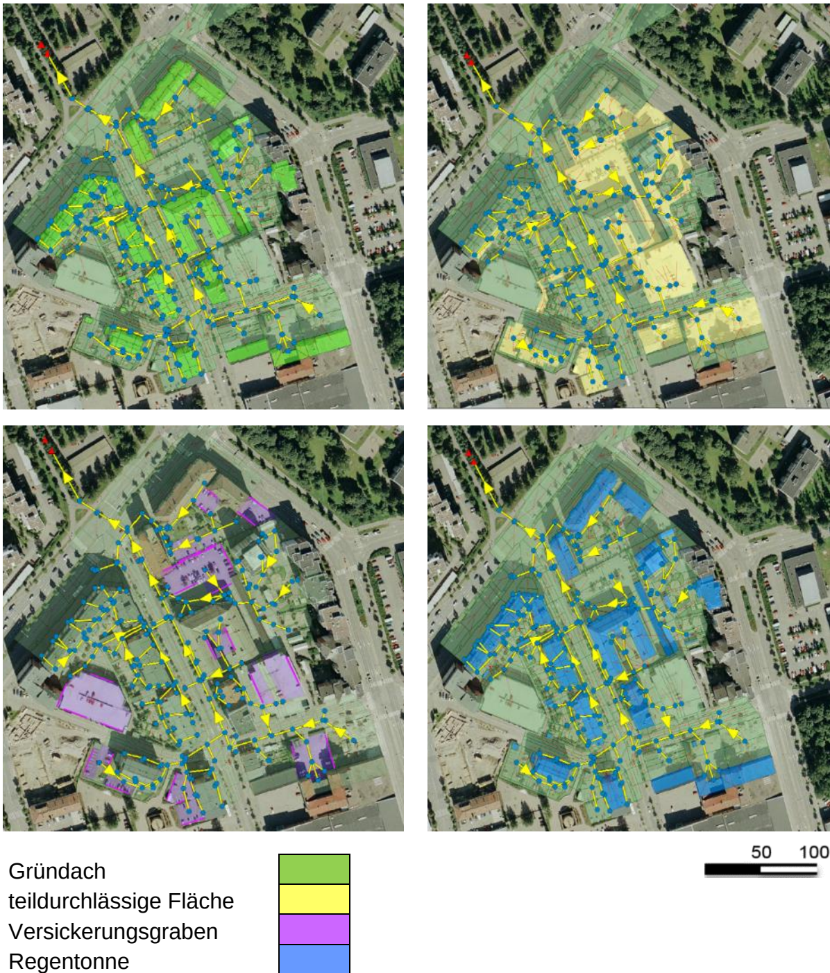
Abbildung 6-1: über LIDs entwässerte Teileinzugsflächen im Einzugsgebiet 1, links oben : Gründach, rechts oben : teildurchlässige Flächen, links unten : Versickerungsgraben, rechts unten : Regentonnen
