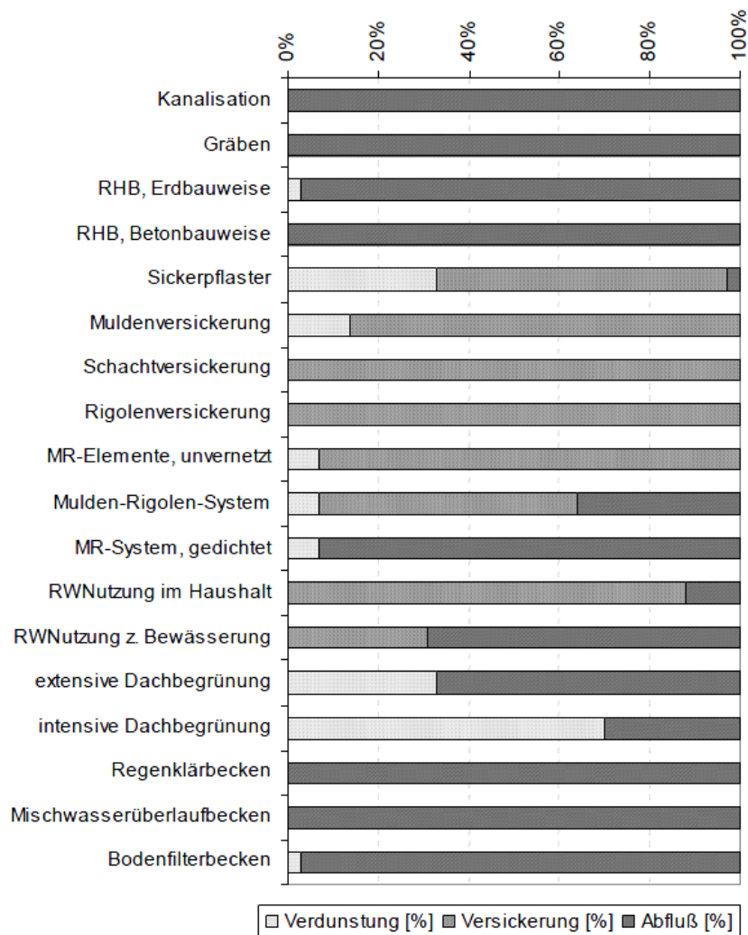
Abbildung 4-8: Wirkung naturnaher Regenwasserbewirtschaftungsanlagen und konventioneller Entwässerung auf den Wasserhaushalt (Sieker, et al., 2009)
