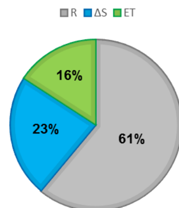
Abbildung 6-4: Wasserbilanzaufstellung in [mm] und in [%] im Ursprungszustand und im adaptierten Zustand im Einzugsgebiet 1
