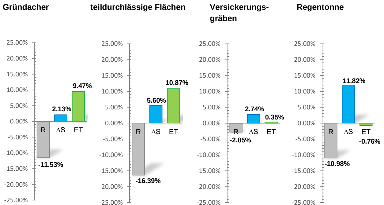
Abbildung 6-5: Änderung der prozentualen Wasserbilanzkomponenten im Einzugsgebiet 1
