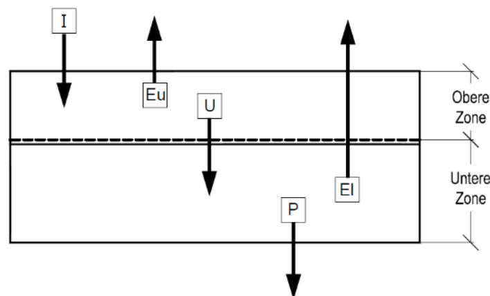
Abbildung 5-8: Grundwasserkörper in PCSWMM; unterteilt in obere (ungesättigt) und untere (gesättigt) Zone (modifiziert nach (Rossman and Huber, 2016))
