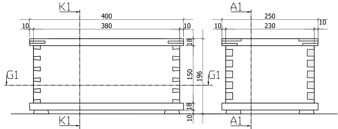
ÜBERSICHTSZEICHNUNG
