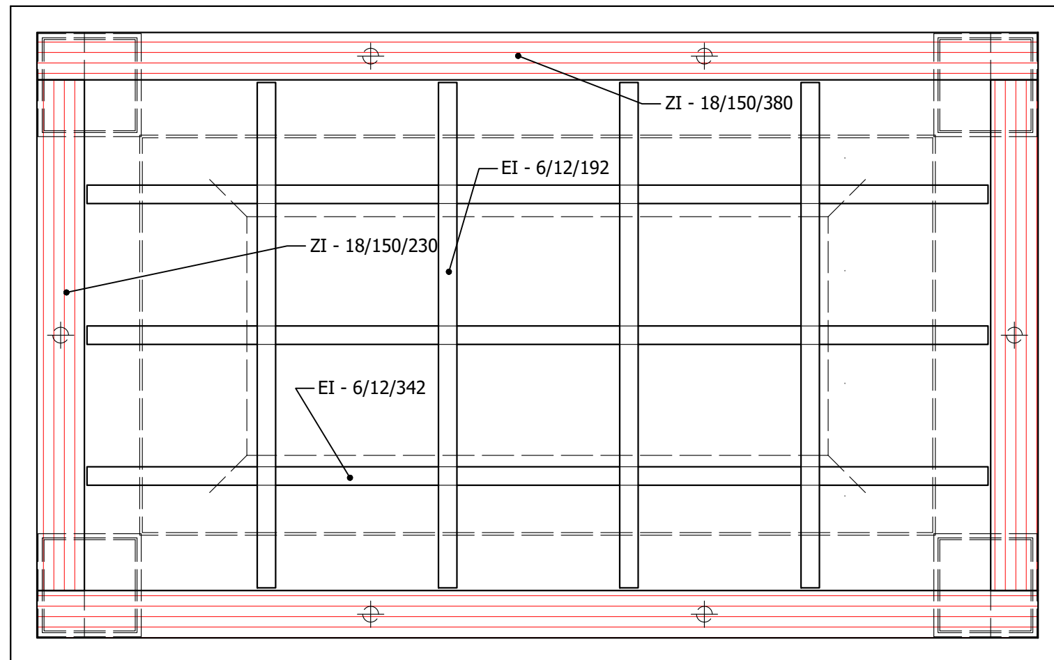
SCHNITT G1
