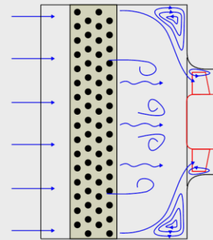
Abb.: Strömungsverhältnisse in der Verdampfer/Ventilator-Einheit einer Außenluft-Wärmepumpe (Bildquelle: Czzielong)
