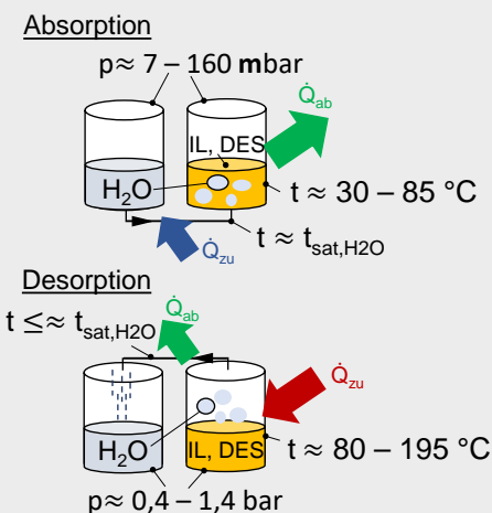
Abb. 2. Vereinfachtes Schema einer möglichen Konstruktion des Versuchsstands inkl. Betriebsbereiche
