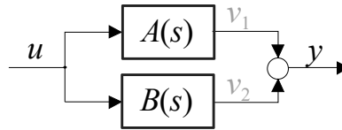
Bild 5.8: Parallelschaltung von Übertragungssystemen
