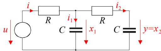
Bild 5.12: Netzwerk, bestehend aus zwei RC-Tiefpass-Schaltungen erster Ordnung
