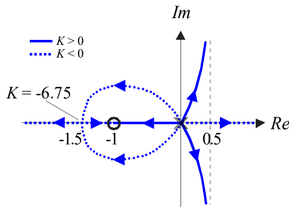
Bild 8.6: Wurzelortskurve zu (8.18)
