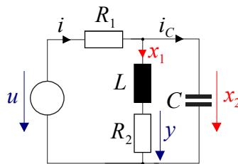
Bild 1.7: Elektrisches Netzwerk mit zwei Energiespeichern
