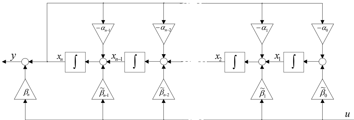
Bild 5.3: Strukturbild zur zweiten Normalform, wobei \tilde{\beta}_i := \beta_i - \alpha_i \beta_n gilt
