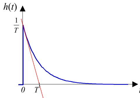
Bild 5.15: Sprungantwort DT 1 -Glieder
