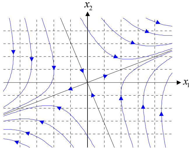
Bild 2.2: Trajektorien zu (2.30) - man spricht in diesem Zusammenhang von einem (instabilen) Sattelpunkt
