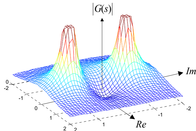
Bild 5.4: Graphische Darstellung von |G(s)| über der komplexen s -Ebene zur Illustration von Pol- und Nullstellen.
