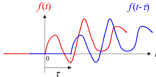
Bild A.1: zur Illustration des Verschiebungssatzes
