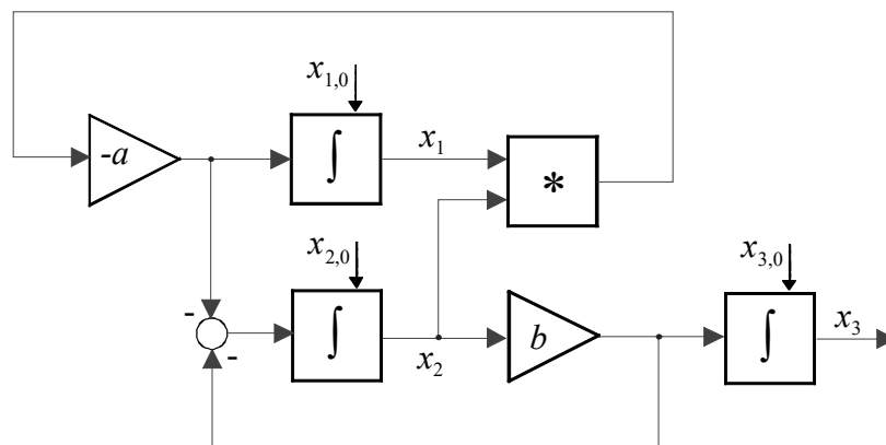
Bild 1.12: Strukturbild zum Epidemiemodell
