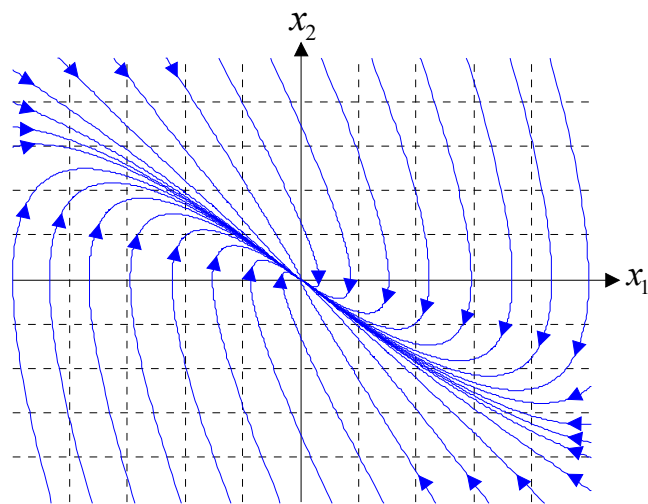
Bild 2.3: Trajektorien zu (2.31) - man spricht in diesem Zusammenhang auch von einem stabilen Knoten
