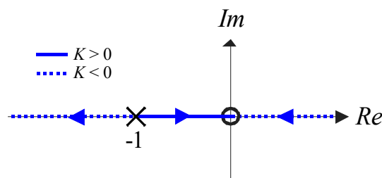
Bild 8.4: Wurzelortskurve zu (8.16)
