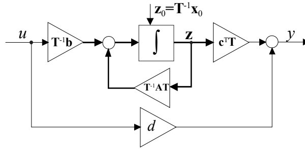
Bild 3.1: Strukturbild des transformierten Systems (3.2)
