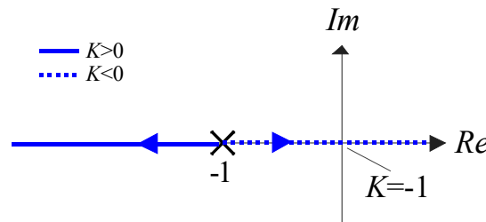
Bild 8.3: Wurzelortskurve zu (8.15)
