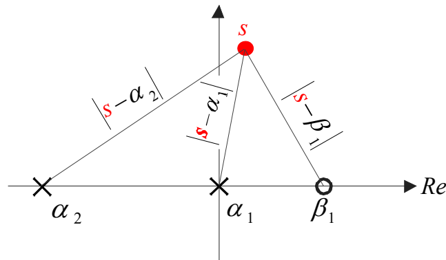
Bild 8.2: Zur Ermittlung von |K| zu einem Punkt s der Wurzelortskurve mittels (8.7)
