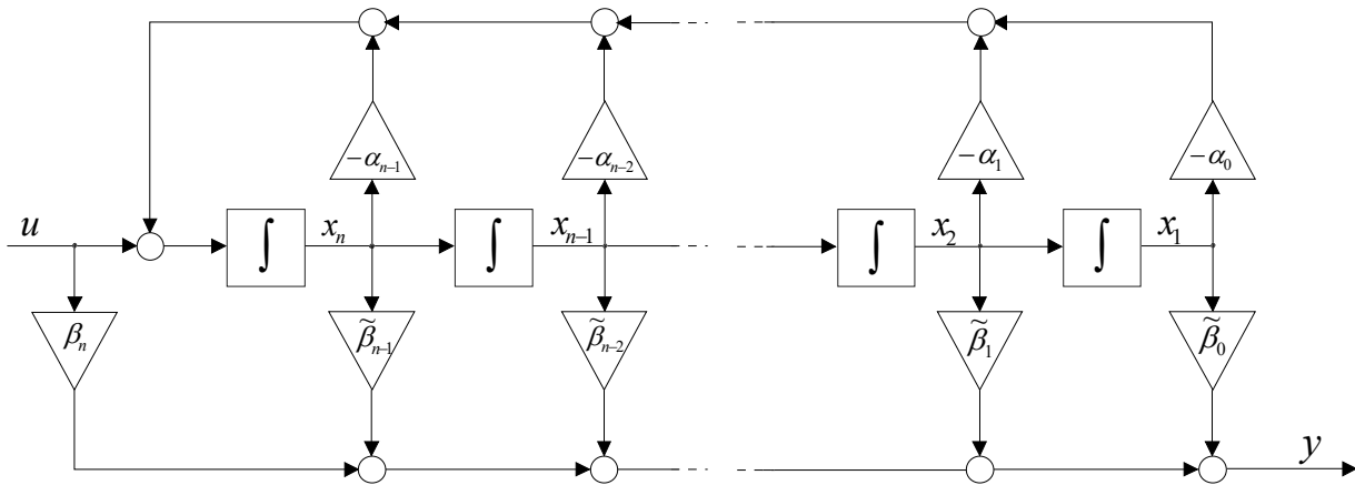
Bild 5.2: Strukturbild zur ersten Normalform, wobei \tilde{\beta}_i := \beta_i - \alpha_i \beta_n gilt
