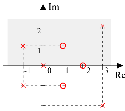
Bild 5.5: PN-Plan zu der Übertragungsfunktion (5.22)
