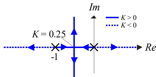
Bild 8.5: Wurzelortskurve zu (8.17)
