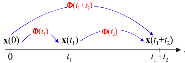
Bild 2.1: Bedeutung der Transitionsmatrix
