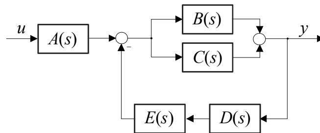
Bild 5.11: Zusammenschaltung mehrerer Übertragungsfunktionen
