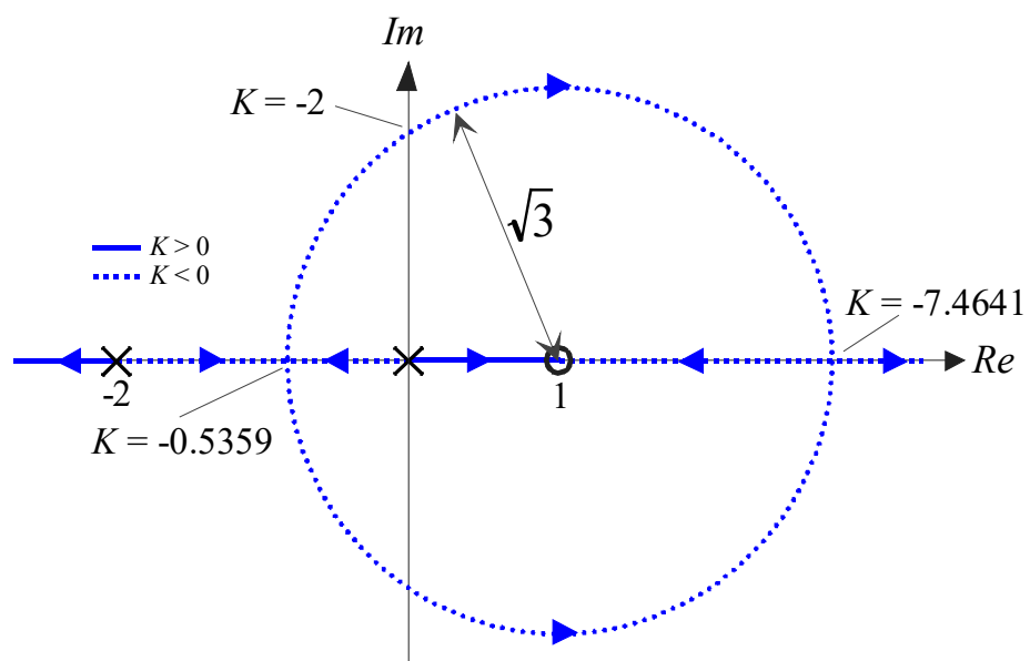
Bild 8.7: Wurzelortskurve zu (8.20)
