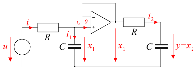
Bild 5.13: Modifikation des Schaltung durch Einbau eines Spannungsfolgers
