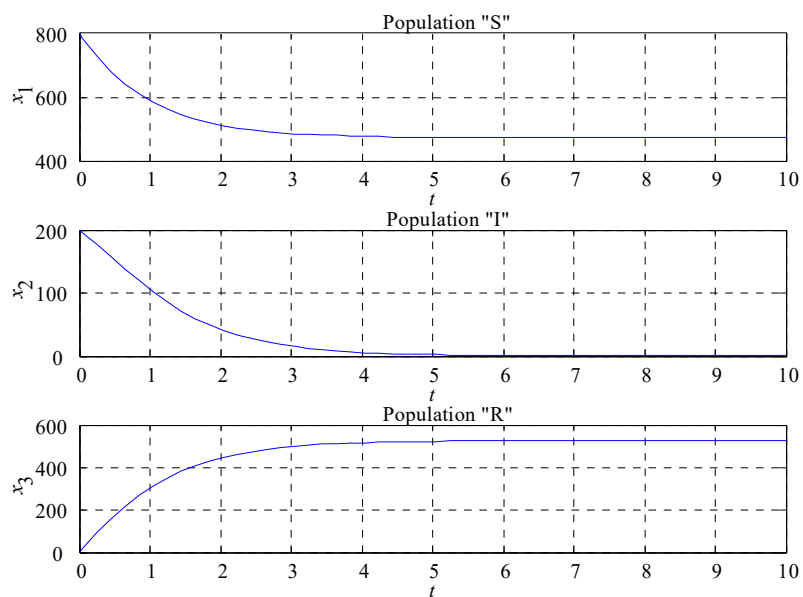
Bild 1.13: Krankheitsverlauf ohne Epidemie
