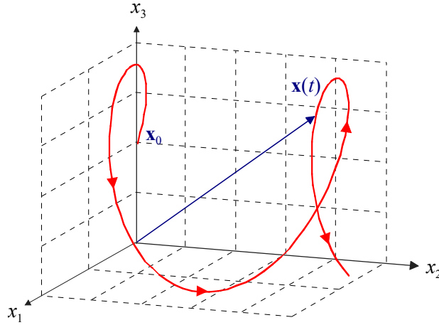
Bild 1.3: Trajektorie im dreidimensionalen Zustandsraum
