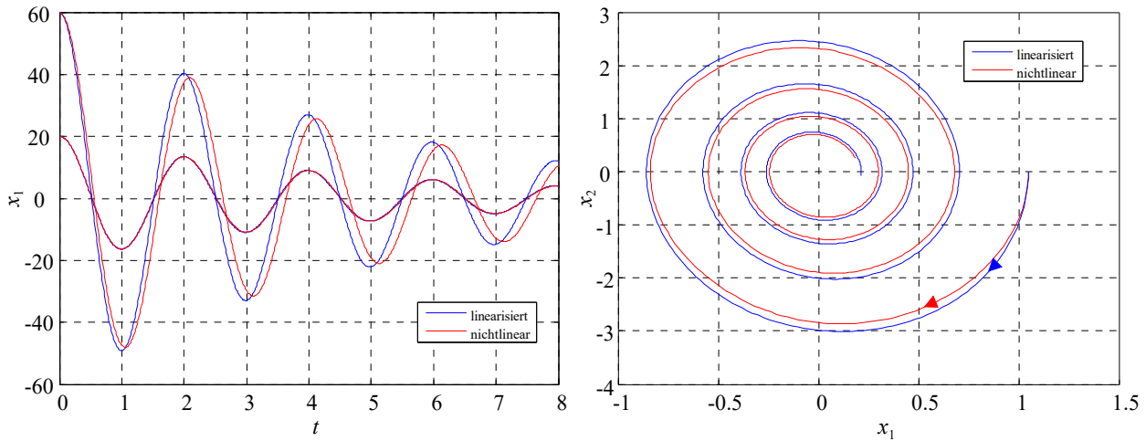
Bild 1.5: Gegenüberstellung des linearisierten Pendelmodells und des nichtlinearen Modells (rot). linkes Bild: Pendelwinkel über Zeit, rechtes Bild: Verlauf der Trajektorien
