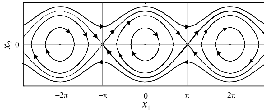
Bild 1.9: Trajektorien des Pendelmodells für k = 0
