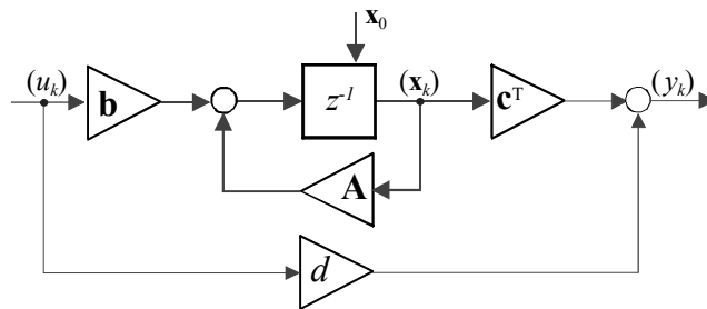
Bild 1.6: Strukturbild eines zeitdiskreten Zustandsmodells der Form (1.22)
