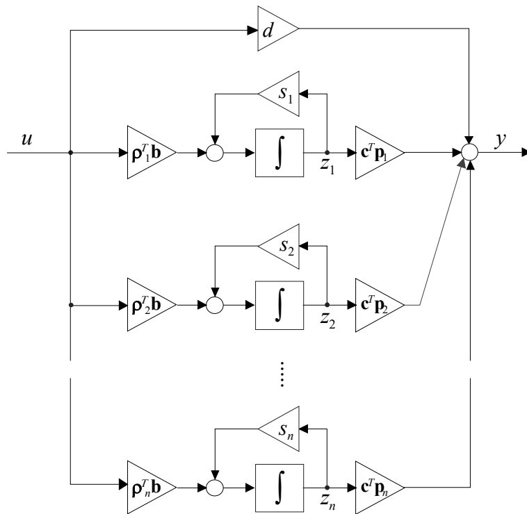
Bild 3.2: Struktur der Diagonalform
