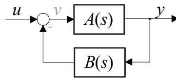
Bild 5.9: Rückgekoppelte Struktur
