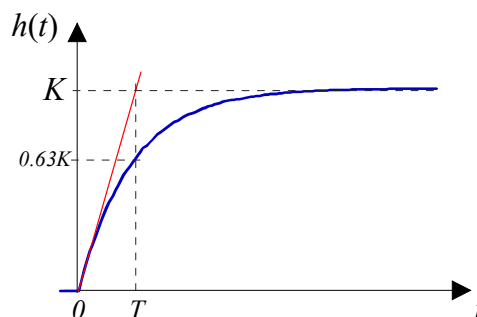
Bild 5.14: Sprungantwort eines PT 1 Elementes mit der Zeitkonstante T
