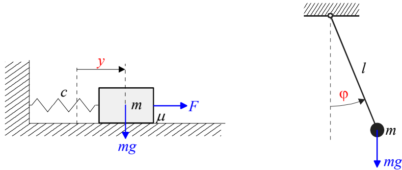
Bild 1.8: Mechanische Systeme: Masse-Feder System und Pendel
