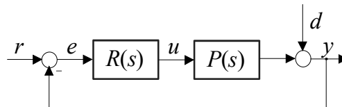
Bild 5.1: Standardregelkreis
