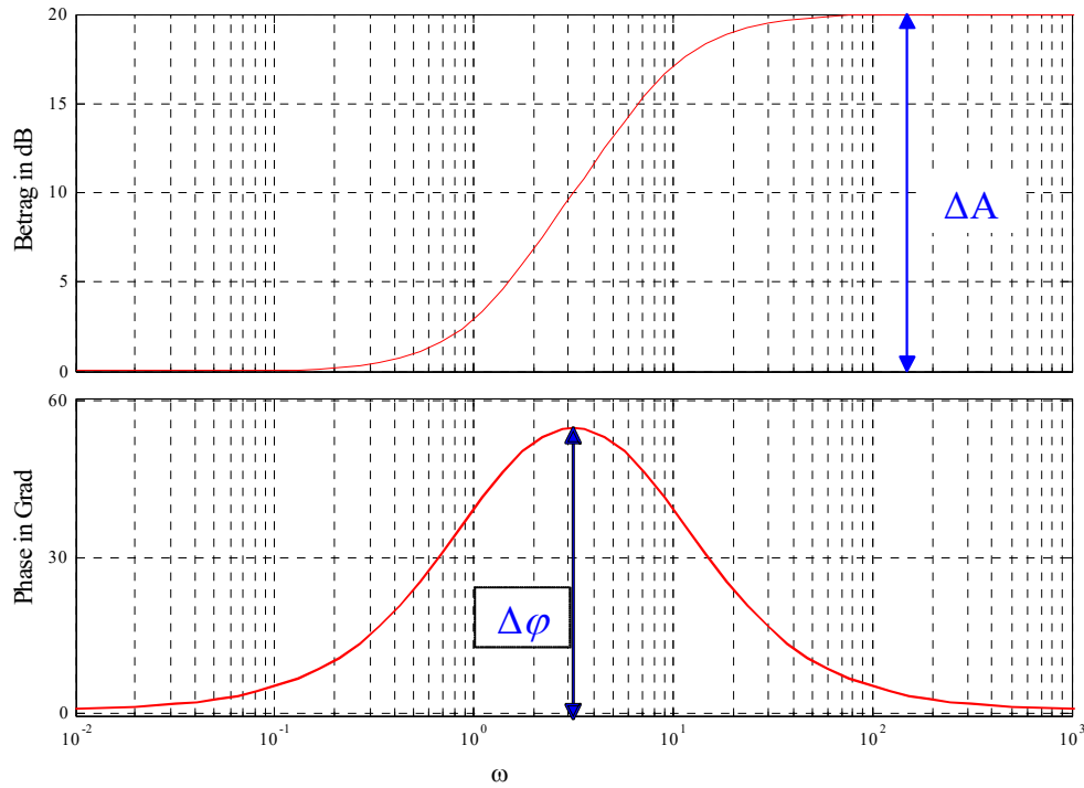
Bild 5.5: Frequenzkennlinien, Lead-Glied
