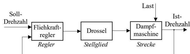
Bild 1.4: Drehzahlregelkreis mit Fliehkraftregler
