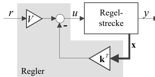
Bild 6.2: Prinzip der Nachführung
