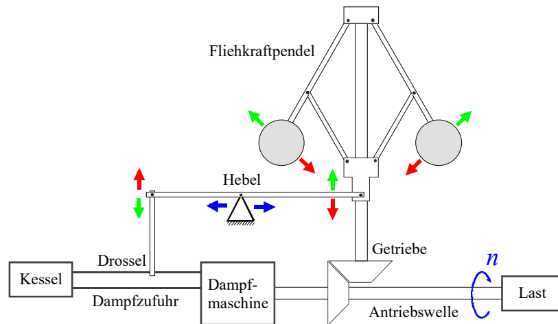
Bild 1.4: Drehzahlregelkreis mit Fliehkraftregler
