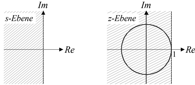
Bild 8.5: Abbildung von \text{Re}\{s\} \leq 0 auf \text{Re}\{z\} \leq 1 bei der Vorwärts-Euler-Integration
