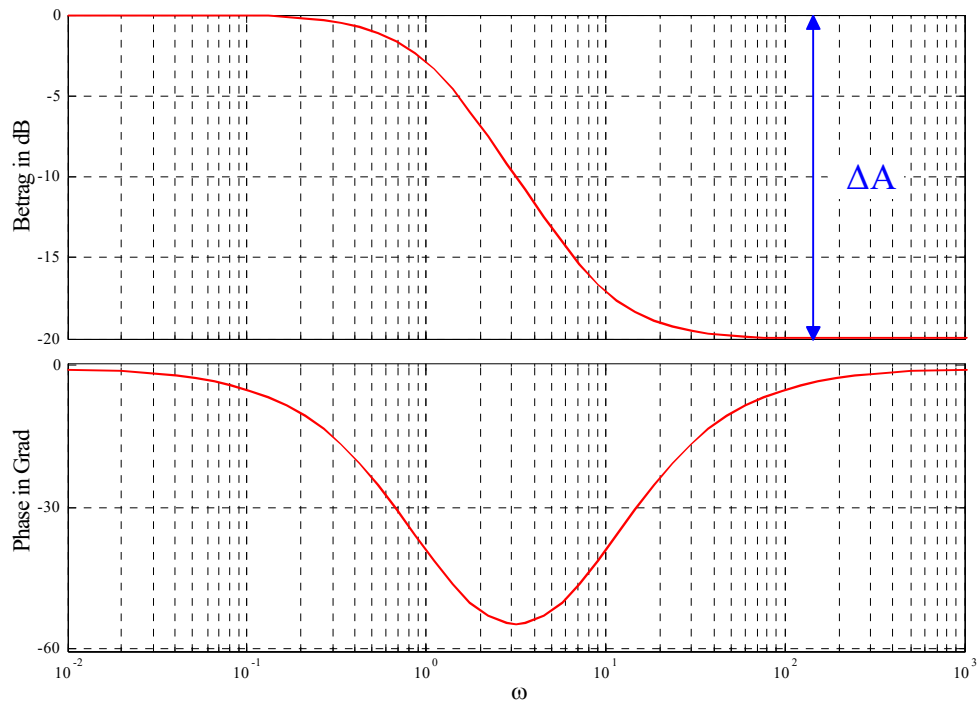
Bild 3.6: Frequenzkennlinien, Lag-Glied
