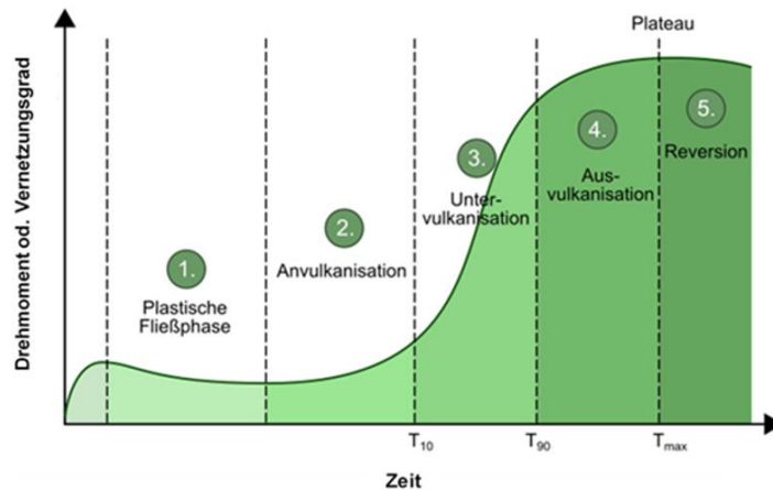
Abb. 6 Typische Vulkanisationskurve (Drehmoment vs. Zeit) mit charakteristischem Verlauf. [12]
