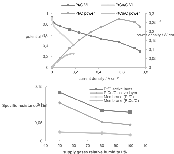
Abb. 2: Polarisationskurven der Hergestellten Elektroden mit 0.4 \text{ mg}_{\text{Pt}} \text{ cm}^{-2} a) und spezifischer Widerstand der Aktivschichten für Protonenleitung b).
