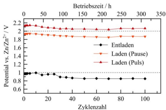
Abb. 4: Gesamte Verlauf der Langzeitmessung einer 60 cm 2 großen Lufterlektrode über insgesamt 100 Zyklen und 300 h.
