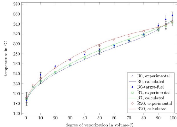
Abb. 2: Siedekurve ASTM D86 (äquivalent zu EN ISO 3405) von Dieseldieselkraftstoff mit 0% (B0), 7% (B7) und 20% (B20) Biodieselanteil, zur Veranschaulichung der Änderung des Siedeverhaltens mit zunehmender Biodiesel-Beimischung.
