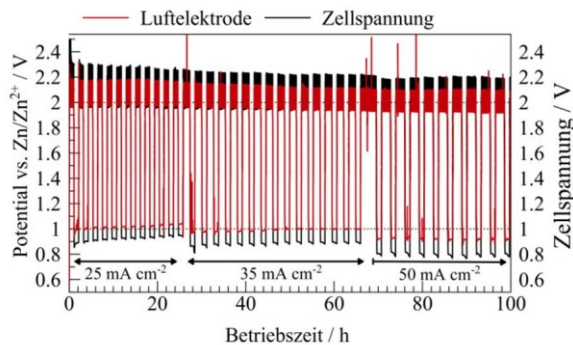
Abb. 3: Die ersten hundert Stunden einer Langzeitmessung einer 60 cm 2 großen Lufterlektrode im Fließzellenbetrieb mit einer Zinkplatte als Gegenelektrode.
