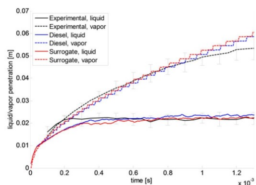
Abb. 3: Ergebnisse von CFD-Simulationen für das Dampf-flüssig-Sprayverhalten eines Dieseldieselkraftstoffs.
