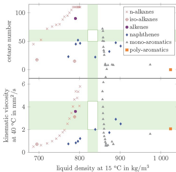
Abb. 1: Dichte, kinematische Viskosität und Cetanzahl typischer Kraftstoffkomponenten zusammen mit den zugehörigen Spezifikationen für Europäische Dieseldieselkraftstoffe (grün hinterlegt). Der mittlere Bereich kennzeichnet den für beide Eigenschaften nach DIN EN 590 simultan zu erfüllenden Bereich. Dieser muss vom resultierenden Surrogat getroffen werden.
