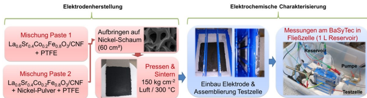
Abb. 2: Herstellung der Luftpolektroden (linke Hälfte) und Aufbau der Fließzelle zur elektrochemischen Charakterisierung (rechte Hälfte).
