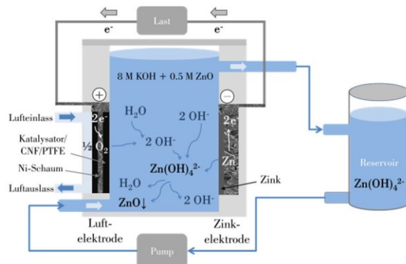
Abb. 1: Schematische Darstellung einer Zink-Luft Fließbatterie: links der Aufbau der Luftelektrode, rechts der Zinkelektrode. Beim Entladen der Batterie wird Zinkat ( \text{Zn(OH)}_4^{2-} ) gebildet, welches in einem externen Tank (Reservoir) gespeichert wird.
