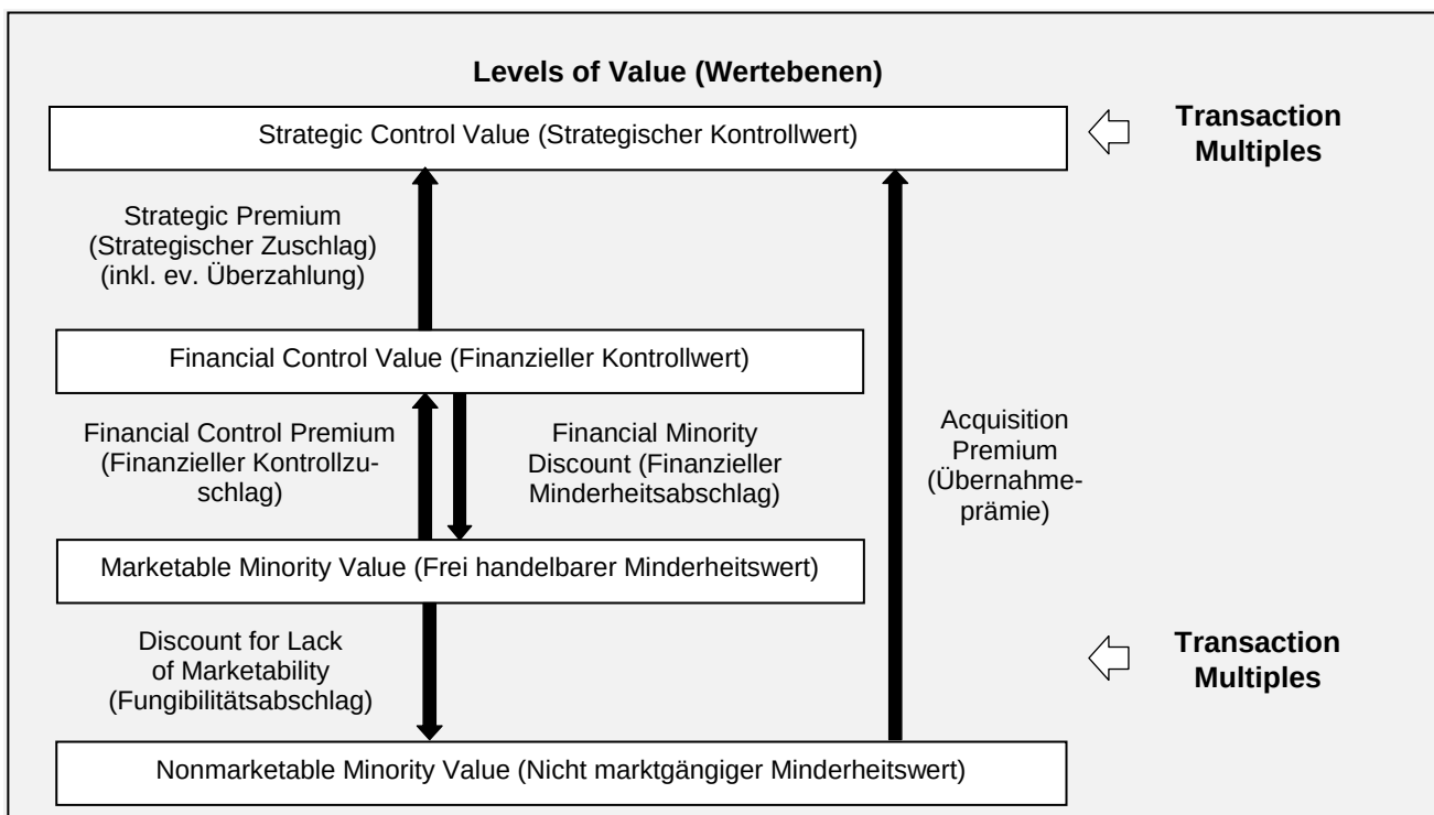
Abbildung 2: Wertebenenmodell
