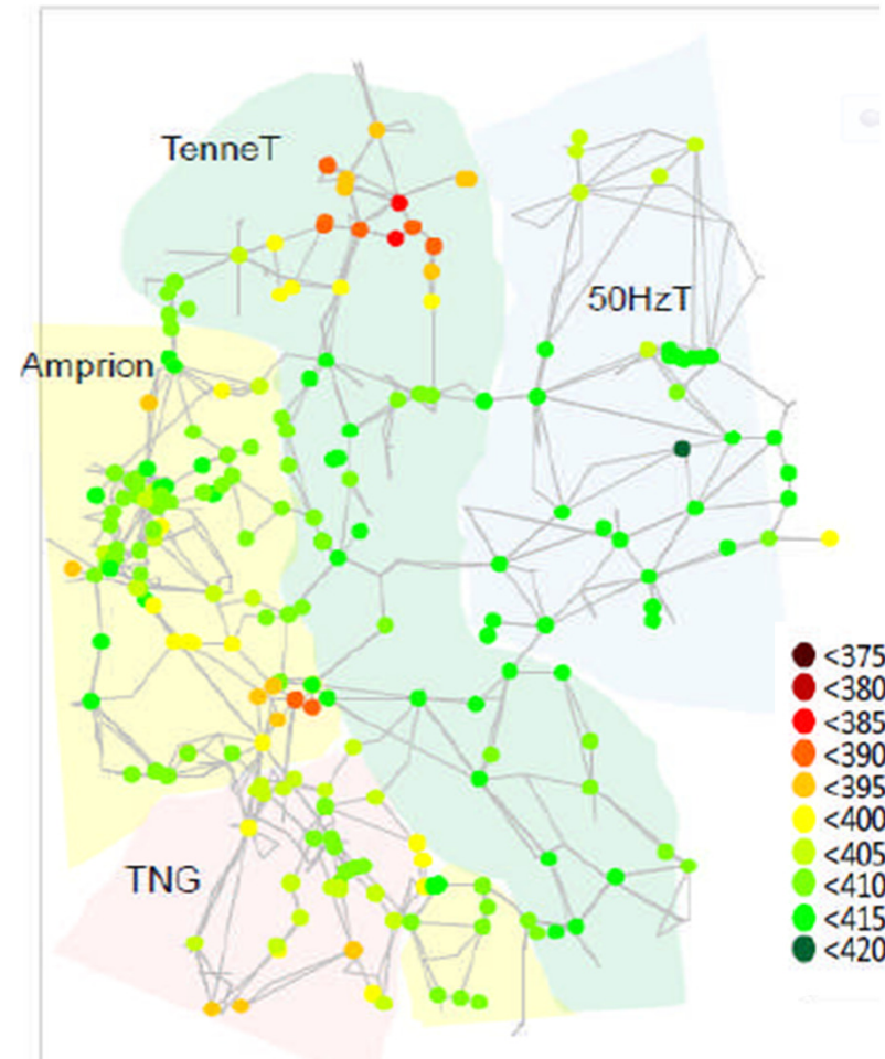
Beispiel für ein Spannungsprofil bei Nichtverfügbarkeit eines AKWs (Quelle: Bericht BNetzA)
